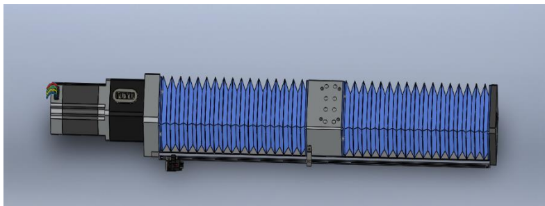
FSK80-BC 电机直连
